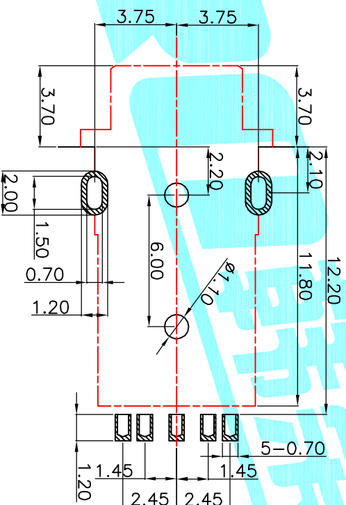
P.C.B Layout
